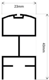
Secțiune profil
